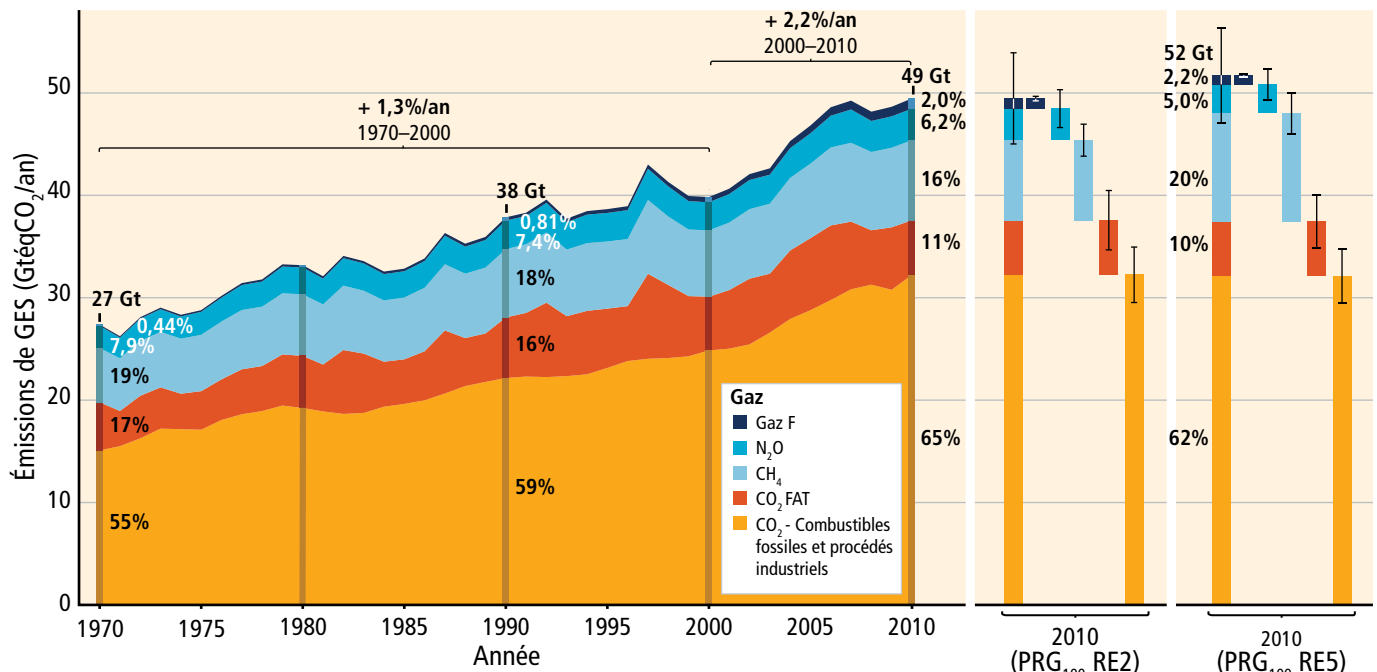
Figure 1.6 | Total annuel des émissions anthropiques de GES (gigatonnes d'équivalent- \text{CO}_2 par an, Gt eq \text{CO}_2 /an) entre 1970 et 2010, par gaz : \text{CO}_2 issu de la combustion de combustibles fossiles et des processus industriels ; \text{CO}_2 issu de la FAT (foresterie et autres affectations des terres) ; méthane ( \text{CH}_4 ) ; oxyde nitreux ( \text{N}_2\text{O} ) ; gaz fluorés (gaz F) réglementés en vertu du Protocole de Kyoto. À droite, émissions en 2010 avec une pondération en équivalent- \text{CO}_2 fondée sur les valeurs figurant dans le deuxième Rapport d'évaluation (RE2) et dans le cinquième Rapport d'évaluation (RE5) du GIEC. Sauf indication contraire, les émissions en équivalent- \text{CO}_2 données dans le présent rapport comprennent la liste des gaz visés par le Protocole de Kyoto ( \text{CO}_2 , \text{CH}_4 , \text{N}_2\text{O} , ainsi que les gaz fluorés) et sont calculées sur la base des valeurs du potentiel de réchauffement global à 100 ans ( \text{PRG}_{100} ) figurant dans le RE2 (voir le glossaire). L'emploi des valeurs de \text{PRG}_{100} plus récentes tirées du RE5 (barres de droite) se traduit par un total annuel plus élevé des émissions de GES (52 Gt eq \text{CO}_2 /an) en raison d'une hausse de la contribution du méthane, sans que la tendance à long terme en soit sensiblement modifiée. D'autres choix modifieraient la contribution des différents gaz (voir l'encadré 3.2). Les valeurs de 2010 sont reprises, par composant, avec les incertitudes correspondantes (intervalle de confiance à 90 %) indiquées par les segments d'erreur. Les émissions mondiales de \text{CO}_2 provenant de l'utilisation de combustibles fossiles sont déterminées avec une marge d'incertitude de 8 % (intervalle de confiance à 90 %). De très grandes incertitudes, de l'ordre de \pm 50 %, sont associées aux émissions de \text{CO}_2 provenant de la FAT. Les incertitudes liées aux émissions mondiales de \text{CH}_4 , de \text{N}_2\text{O} et de gaz F sont estimées respectivement à 20 %, 60 % et 20 %. L'année 2010 est l'année la plus récente pour laquelle des statistiques sur les émissions de tous les gaz ainsi que l'évaluation des incertitudes étaient quasi complètes à la date limite fixée pour la rédaction du rapport. Les incertitudes estimées concernent uniquement les émissions, elles ne rendent pas compte de l'incertitude touchant les PRG (selon la section 8.7 du rapport du GT I). {GT III figure RID.1}
