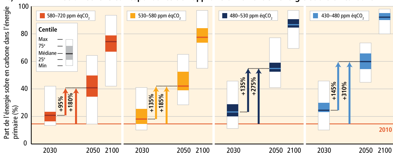
Figure 3.2 | a) Émissions mondiales de gaz à effet de serre (en gigatonnes d'équivalent- \text{CO}_2 par an (GtEq \text{CO}_2 /an)) pour différents niveaux de concentration à long terme, et b) exigences d'une mise à l'échelle correspondante de l'approvisionnement en énergie sobre en carbone (pourcentage de l'énergie primaire) pour 2030, 2050 et 2100 par rapport aux niveaux de 2010 dans les scénarios d'atténuation. [GT III RID.4, figure 6.7, figure 7.16] [Note: les émissions d'éq-GtCO 2 prennent en compte la liste des gaz régis par le Protocole de Kyoto (dioxyde de carbone ( \text{CO}_2 ), méthane ( \text{CH}_4 ), oxyde nitreux ( \text{N}_2\text{O} ) et gaz fluorés). Elles sont calculées en fonction de leur potentiel de réchauffement global sur 100 ans (PRG 100 ), dont les valeurs ont été établies dans le deuxième Rapport d'évaluation du GIEC.]
