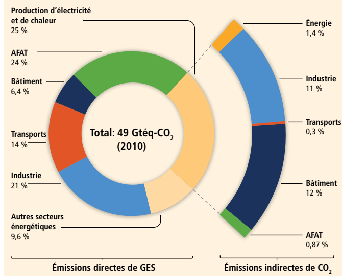
Figure 1.7 | Répartition des émissions anthropiques totales de GES (gigatonnes d'équivalent-CO 2 par an, Gtéc CO 2 /an) entre les secteurs économiques en 2010. La couronne montre les parts (en pourcentage des émissions anthropiques totales de GES) des émissions directes de GES attribuées en 2010 à cinq secteurs économiques. L'arc agrandi sur la droite indique la répartition (en pourcentage des émissions anthropiques totales de GES) des émissions indirectes de CO 2 découlant de la production d'électricité et de chaleur entre les secteurs qui consomment l'énergie finale. La part attribuée aux «autres secteurs énergétiques» correspond à toutes les sources d'émission de GES dans le secteur de l'énergie, comme il est défini dans l'annexe II du rapport du GT III, mis à part la production d'électricité et de chaleur [GT III annexe II.9.1]. Les données relatives à l'AFAT (agriculture, foresterie et autres affectations des terres) incluent les émissions de CO 2 d'origine terrestre provoquées par les feux de forêt et de tourbière ainsi que par la décomposition dans les tourbières; elles se rapprochent des flux nets de CO 2 attribués à la FAT (foresterie et autres affectations des terres), que décrit le chapitre 11 du rapport du GT III. Toutes les émissions sont exprimées en Gtéc CO 2 sur la base du potentiel de réchauffement global à 100 ans (PRG 100 ) figurant dans le deuxième Rapport d'évaluation du GIEC (RE2). Les secteurs sont définis dans l'annexe II.9 du rapport du GT III. [GT III figure RID.2]
