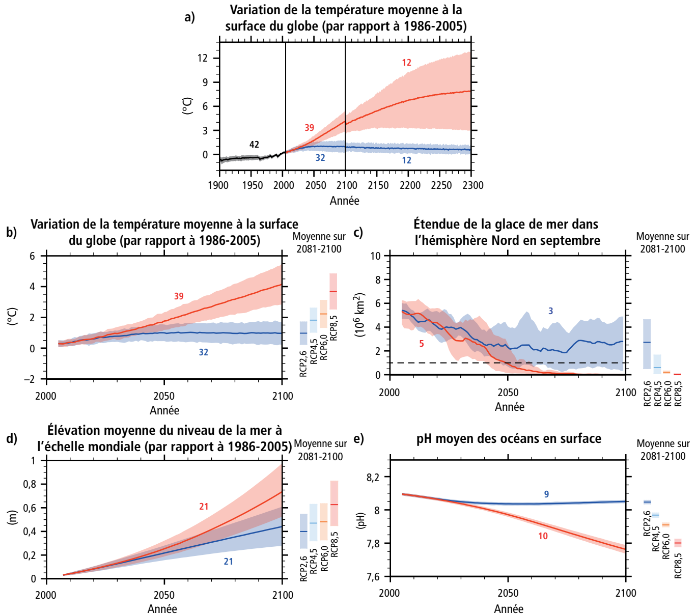
Figure 2.1 | a) Série chronologique des variations de la température moyenne à la surface du globe entre 1900 et 2300 (par rapport à la période 1986–2005), établie à partir d'expériences de la cinquième phase de l'exercice de comparaison de modèles couplés (CMIP5) axées sur les concentrations. Les projections sont indiquées pour la moyenne multimodèle (traits pleins) et la fourchette de 5 à 95 % pour la distribution des modèles individuels (zone ombrée). Les lignes grises et les zones ombrées représentent les simulations historiques de la CMIP5. Les discontinuités prévues pour 2100, dues au fait que différents modèles prolongent les calculs au-delà du XXI e siècle, n'ont pas de signification physique. b) Identique à a), mais pour la période 2006-2100 (par rapport à la période 1986–2005). c) Étendue de la glace de mer dans l'hémisphère Nord en septembre (moyenne glissante sur 5 ans). La ligne pointillée représente des conditions presque sans glace (c'est-à-dire lorsque l'étendue de glace de mer en septembre est inférieure à 10 6 km 2 pendant au moins cinq années consécutives). d) Variation du niveau moyen de la mer à l'échelle mondiale. e) Variation du pH des océans en surface. Dans tous les cadres, les séries chronologiques des projections et une mesure de l'incertitude (zones ombrées) sont présentées pour les scénarios RCP2,6 (en bleu) et RCP8,5 (en rouge). Le nombre de modèles CMIP5 utilisés pour calculer la moyenne multimodèle est indiqué. Les moyennes et incertitudes associées sur la période 2081-2100 sont fournies pour tous les scénarios RCP sous forme de bandes verticales de couleur situées à droite des cadres b) à e). Pour l'étendue de la glace de mer mentionnée en c), la prévision de moyenne et d'incertitude (plage minimum-maximum) n'est donnée que pour le sous-ensemble de modèles qui reproduisent le plus fidèlement la moyenne climatologique et l'évolution de la glace de mer arctique pour la période 1979-2012. Pour le niveau de la mer illustré en d), en l'état actuel des connaissances (découlant d'observations, de la compréhension des causes physiques et de modélisations), seul l'effondrement de secteurs marins de la nappe glaciaire de l'Antarctique, si celui-ci était provoqué, pourrait faire monter de manière importante le niveau moyen de la mer au-dessus de la plage probable des valeurs au cours du XXI e siècle. Cependant, cette contribution supplémentaire ne dépasserait pas quelques dixièmes de mètre d'élévation du niveau de la mer au cours du XXI e siècle ( degré de confiance moyen ). [GT I figure RID.7, figure RID.9, figure 12.5, 6.4.4, 12.4.1, 13.4.4, 13.5.1]
