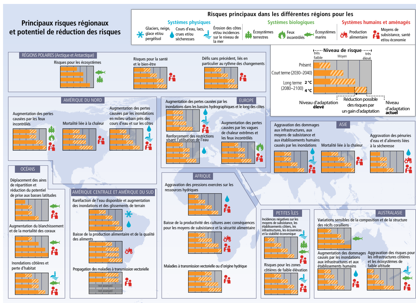
Figure 2.4 | Risques principaux représentatifs de chaque région. Ce graphique indique aussi les options envisageables pour réduire ces risques grâce à des mesures d'adaptation et d'atténuation, ainsi que les limites de l'adaptation. La détermination des risques principaux s'appuie sur des avis d'experts et sur les critères particuliers suivants: grande ampleur, forte probabilité ou irréversibilité des incidences; chronologie des incidences; vulnérabilité ou exposition persistantes; possibilités limitées de réduire les risques par des mesures d'adaptation ou d'atténuation. Les niveaux de risque peuvent être très faibles, faibles, moyens, élevés ou très élevés à trois horizons temporels: le présent, à court terme (en l'occurrence, 2030–2040) et à long terme (2080–2100). À court terme, les niveaux prévus d'augmentation de la température moyenne à l'échelle du globe ne divergent pas beaucoup d'un scénario d'émissions à l'autre. À long terme, les niveaux de risque sont analysés selon deux scénarios possibles (augmentation de la température moyenne à l'échelle du globe de 2 ou 4 °C par rapport aux niveaux préindustriels). Pour chaque horizon temporel, les niveaux de risque sont indiqués sur la base d'une poursuite de l'adaptation actuelle et en faisant l'hypothèse de niveaux élevés d'adaptation actuelle et future. Les niveaux de risque ne sont pas nécessairement comparables, notamment d'une région à l'autre. {GT II RID encadré d'évaluation RID.2 tableau 1}
