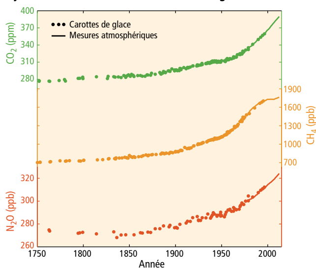
Moyennes mondiales des concentrations de gaz à effet de serre
