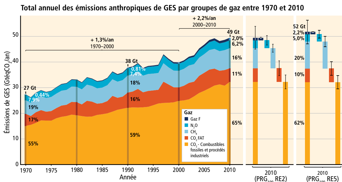
Figure RID.2 | Total annuel des émissions anthropiques de gaz à effet de serre (GES) (gigatonne d'équivalent CO 2 par an, GtéquCO 2 /an), pour la période 1970–2010 et par gaz : CO 2 issu de l'usage des combustibles fossiles et des procédés industriels; CO 2 issu de la foresterie et d'autres affectations des terres (FAT); méthane (CH 4 ); oxyde nitreux (N 2 O); gaz fluorés (gaz F) réglementés en vertu du protocole de Kyoto. À droite sont représentées côte à côte les émissions de 2010 en équivalent CO 2 , suivant des pondérations établies à partir d'une part des valeurs du deuxième Rapport d'évaluation du GIEC (RE2) et d'autre part des valeurs du cinquième Rapport d'évaluation du GIEC (RE5). Sauf indication contraire, les émissions en équivalent CO 2 dont il est question dans le Rapport de synthèse regroupent tous les gaz réglementés en vertu du protocole de Kyoto (CO 2 , CH 4 , N 2 O et gaz F); elles sont établies à partir des valeurs du potentiel de réchauffement global calculées à un horizon de cent ans (PRG 100 ) tirées du RE2 (voir le glossaire). En se servant des valeurs du PRG 100 les plus récentes, à savoir celles du RE5 (boîtes à moustaches à droite), on obtient un total annuel des émissions de GES plus élevé (52 GtéquCO 2 /an) qu'il faut attribuer à une contribution accrue du méthane, ce qui ne modifie pas beaucoup la tendance à long terme. {figure 1.6, encadré 3.2}
