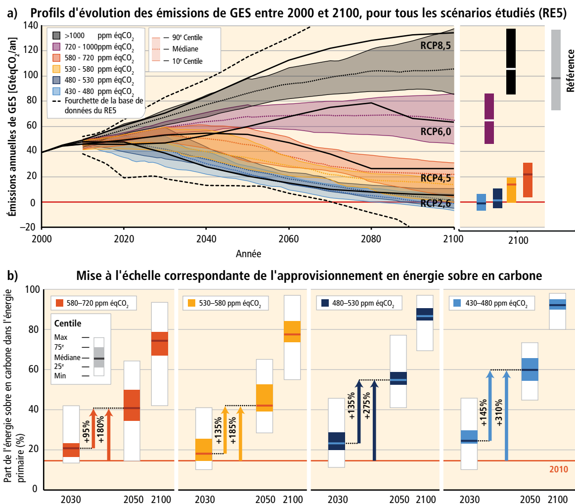
Figure RID.11 | Émissions mondiales de gaz à effet de serre (Gt \text{eqCO}_2/\text{an} ) dans les scénarios de référence et d'atténuation pour différents niveaux de concentration à long terme (a) et exigences d'une mise à l'échelle correspondante de l'approvisionnement en énergie sobre en carbone (pourcentage de l'énergie primaire) pour 2030, 2050 et 2100 par rapport aux niveaux de 2010 dans les scénarios d'atténuation (b) . {figure 3.2}
