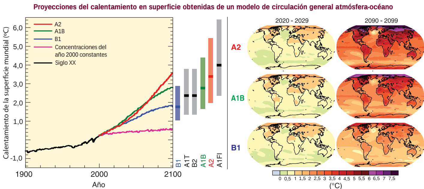
Figura 3.2. Gráfica izquierda: Las líneas de trazo continuo representan promedios mundiales multimodelo del calentamiento en superficie (respecto del periodo 1980-1999) para los escenarios IEEE A2, A1B y B1, representados como continuación de las simulaciones del siglo XX. La línea anaranjada describe un experimento cuyas concentraciones se mantuvieron constantes en valores del año 2000. Las barras del centro de la Figura representan la estimación óptima (línea gruesa transversal interior) y el intervalo de valores probables para los seis escenarios testimoniales IEEE en el periodo 2090-2099 respecto de 1980-1999. La estimación óptima y los intervalos probables representados por las barras abarcan los modelos de circulación general atmósfera-oceano (MCGAO) indicados en la parte izquierda, así como los resultados de una jerarquía de modelos independientes y las limitaciones observacionales.
