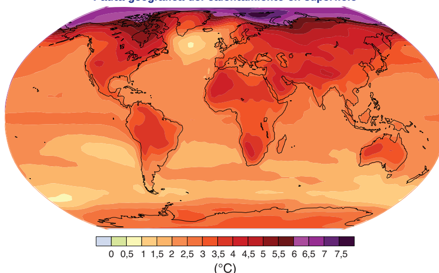
Figura RRP. 6. Cambios de la temperatura superficial proyectados para finales del siglo XXI (2090-2099). Se indica en el mapa la proyección multi-MCGAO promediada para el escenario A1B del IPCC. Todas las temperaturas tienen como referencia el período 1980-1999. {Figura 3.2}
