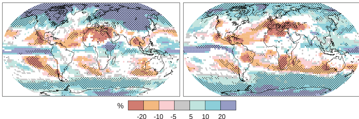
Figura 3.3. Cambios de la precipitación relativos (en valores porcentuales) para el período 2090-2099, respecto del período 1980-1999. Los valores son promedios multimodelo basados en el escenario A1B (IEEE) para los períodos diciembre-febrero (izquierda) y junio-agosto (derecha). Las áreas en blanco representan los lugares en que más de un 66% de los modelos coinciden en el signo del cambio, y las áreas punteadas representan los lugares en que más de un 90% de los modelos concuerdan en el signo del cambio. {GTI Figura 10.9, RRP}
