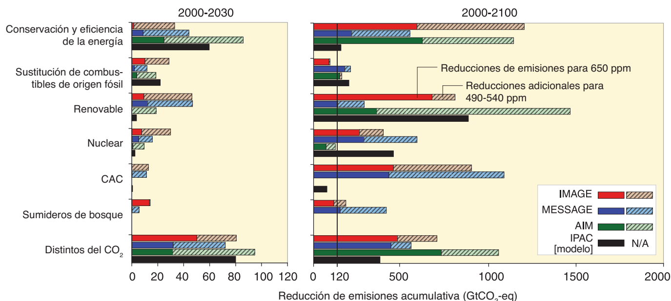
Figura 5.2 Reducciones de emisiones acumulativas resultantes de medidas de mitigación alternativas para el período 2000-2030 (imagen izquierda) y para el 2000-2100 (imagen derecha). En la figura se describen escenarios ilustrativos correspondientes a cuatro modelos (AIM, IMAGE, IPAC y MESSAGE) tendentes a la estabilización en niveles bajos (entre 490 y 540 ppm de CO 2 -eq) e intermedios (650 ppm de CO 2 -eq), respectivamente. Las barras de color oscuro denotan reducciones para un objetivo de 650 ppm de CO 2 -eq, mientras que las barras de color claro denotan las reducciones adicionales necesarias para conseguir el nivel de entre 490 y 540 ppm de CO 2 -eq. Obsérvese que algunos modelos no contemplan medidas de mitigación basadas en la potenciación de los sumideros de los bosques (AIM y IPAC) o en la CAC (AIM), y que la parte que representan las opciones de energías bajas en carbono respecto del suministro de energía total está también determinada por la inclusión de esas opciones en el escenario de referencia. El concepto de CAC abarca la captación y almacenamiento de CO 2 a partir de la biomasa. Los sumideros de bosque incluyen la reducción de emisiones por deforestación. En la figura se describen reducciones de emisiones en escenarios de referencia con unas emisiones acumulativas de entre 6000 y 7000 GtCO 2 -eq (2000-2100). {GTIII Figura RRP.9}
