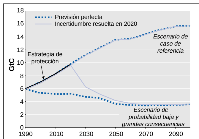
Figura RT-10b: Estrategia óptima de protección para un escenario de probabilidad baja y grandes consecuencias, usando un enfoque de optimización de costo-beneficios.
