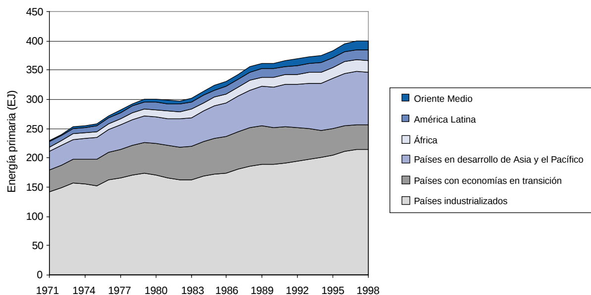
Figura RT-3: Uso mundial de energía primaria por región entre 1971 y 1998.
