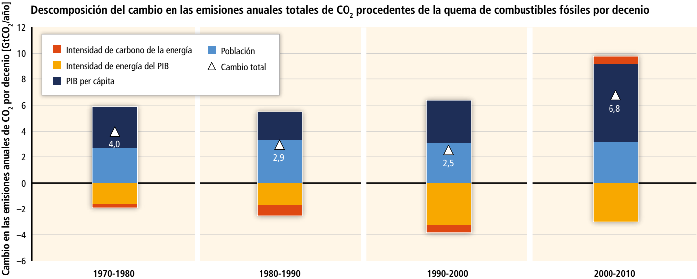
Figura RRP.3 Descomposición del cambio decenal en las emisiones anuales totales de CO 2 procedentes de la quema de combustibles fósiles por cuatro factores impulsores: población, ingreso (PIB) per cápita, intensidad de energía del PIB e intensidad de carbono de la energía. Los segmentos de las barras muestran los cambios asociados con cada factor por separado, manteniendo constantes los demás factores respectivos. Los cambios en las emisiones totales se indican mediante un triángulo. Los cambios en las emisiones a lo largo de cada decenio se miden en gigatoneladas (Gt) de CO 2 por año [GtCO 2 /año]; el ingreso se convierte en unidades comunes utilizando paridades de poder adquisitivo. [figura 1.7]
