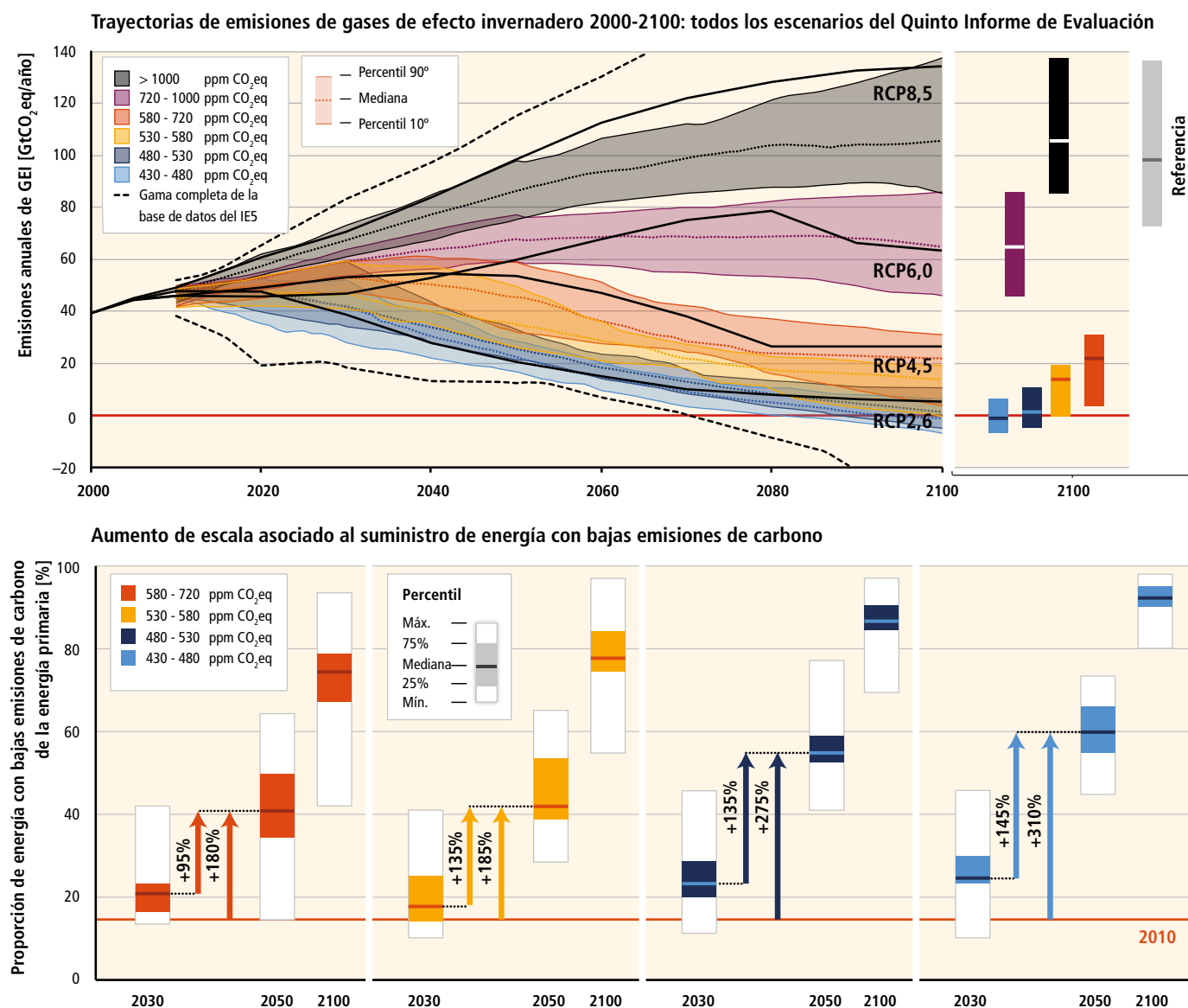
Figura RRP.4 | Trayectorias de las emisiones globales de GEI (GtCO 2 eq/año) en los escenarios de referencia y de mitigación para distintos niveles de concentración a largo plazo (parte superior) [figura 6.7] y requisitos del aumento de escala asociados a la energía con bajas emisiones de carbono (porcentaje de energía primaria) para 2030, 2050 y 2100 en comparación con los niveles de 2010 en los escenarios de mitigación (parte inferior) [figura 7.16]. En el gráfico inferior se excluyen los escenarios con limitada disponibilidad tecnológica y trayectorias exógenas de los precios del carbono. Para las definiciones de emisiones de CO 2 -equivalente y concentraciones de CO 2 -equivalente, véase el Glosario de GTIII IES.
