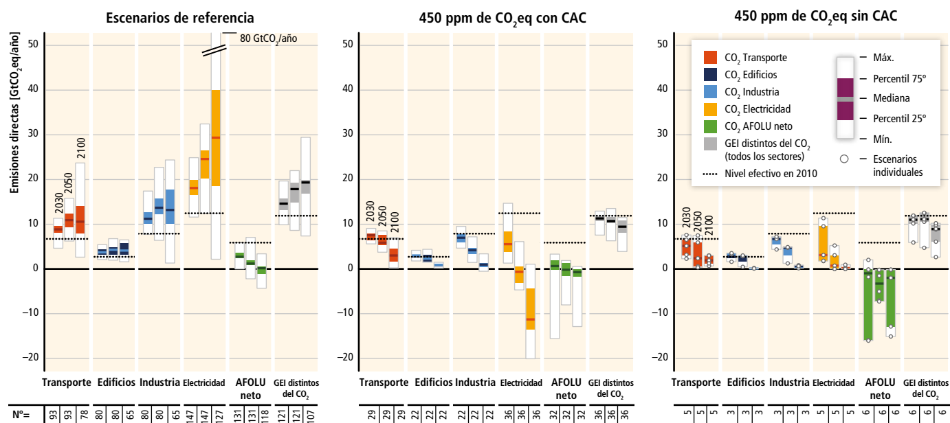
Figura RRP.7 Emisiones directas de CO 2 por sector y GEI distintos del CO 2 totales (gases enumerados en el Protocolo de Kyoto) en los distintos sectores en los escenarios de referencia (gráfico de la izquierda) y en los escenarios de mitigación en los que se llega a aproximadamente 450 (430-480) ppm de CO 2 eq con CAC (gráfico central) y sin CAC (gráfico de la derecha). Los números en la base de los gráficos indican el número de escenarios abarcados en el rango, que difiere entre los sectores y los años debido a las distintas resoluciones sectoriales y horizontes temporales de los modelos. Obsérvese que muchos modelos no pueden llegar a una concentración de aproximadamente 450 ppm de CO 2 eq en 2100 sin CAC, por lo que es menor el número de escenarios del gráfico de la derecha. [figuras 6.34 y 6.35]
