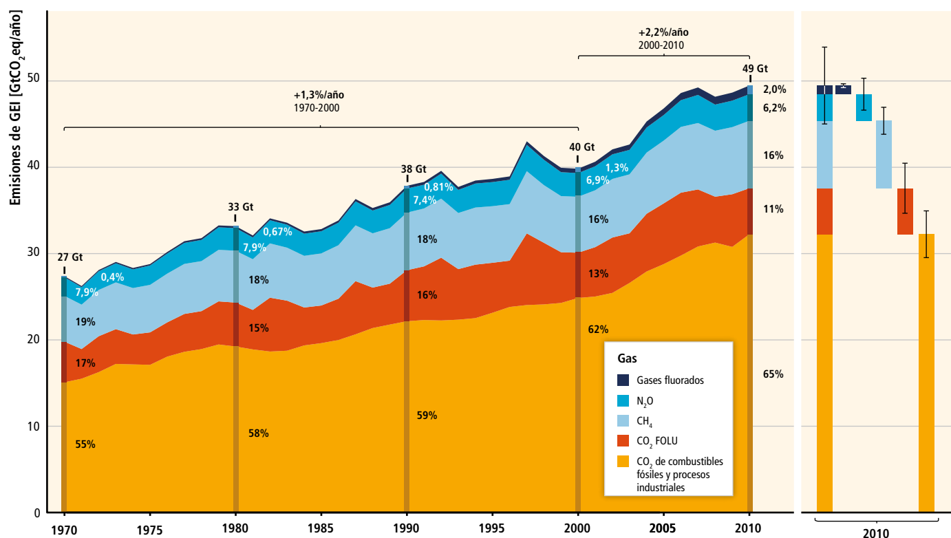
Emisiones antropógenas anuales de GEI totales por grupos de gases, 1970-2010
