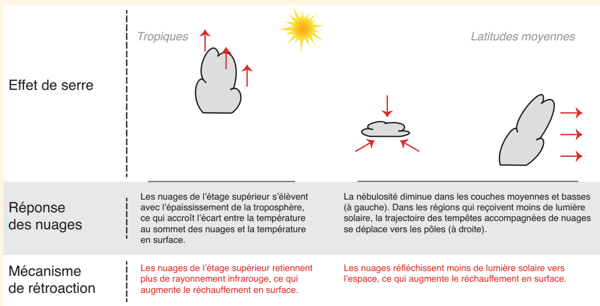
FAQ 7.1 - Figure 1 | Schéma des grands mécanismes de rétroaction nuageuse.
