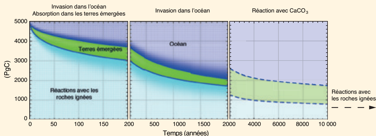
FAQ 6.2 - Figure 2 | Décroissance d'un volume de \text{CO}_2 excédentaire (5 000 PgC) rejeté dans l'atmosphère au moment zéro et sa répartition dans les terres émergées et l'océan en fonction du temps, selon des modèles couplés climat-cycle du carbone. La taille des bandes colorées indique l'absorption de carbone par le réservoir en question. Les deux premiers graphiques correspondent à la moyenne multimodèles issue d'un projet de comparaison de modèles (Joos et al. , 2013). Le dernier montre la redistribution à plus long terme, y compris la dissolution des sédiments carbonatés dans l'océan, selon un modèle du système Terre de complexité intermédiaire (d'après Archer et al. , 2009b).
