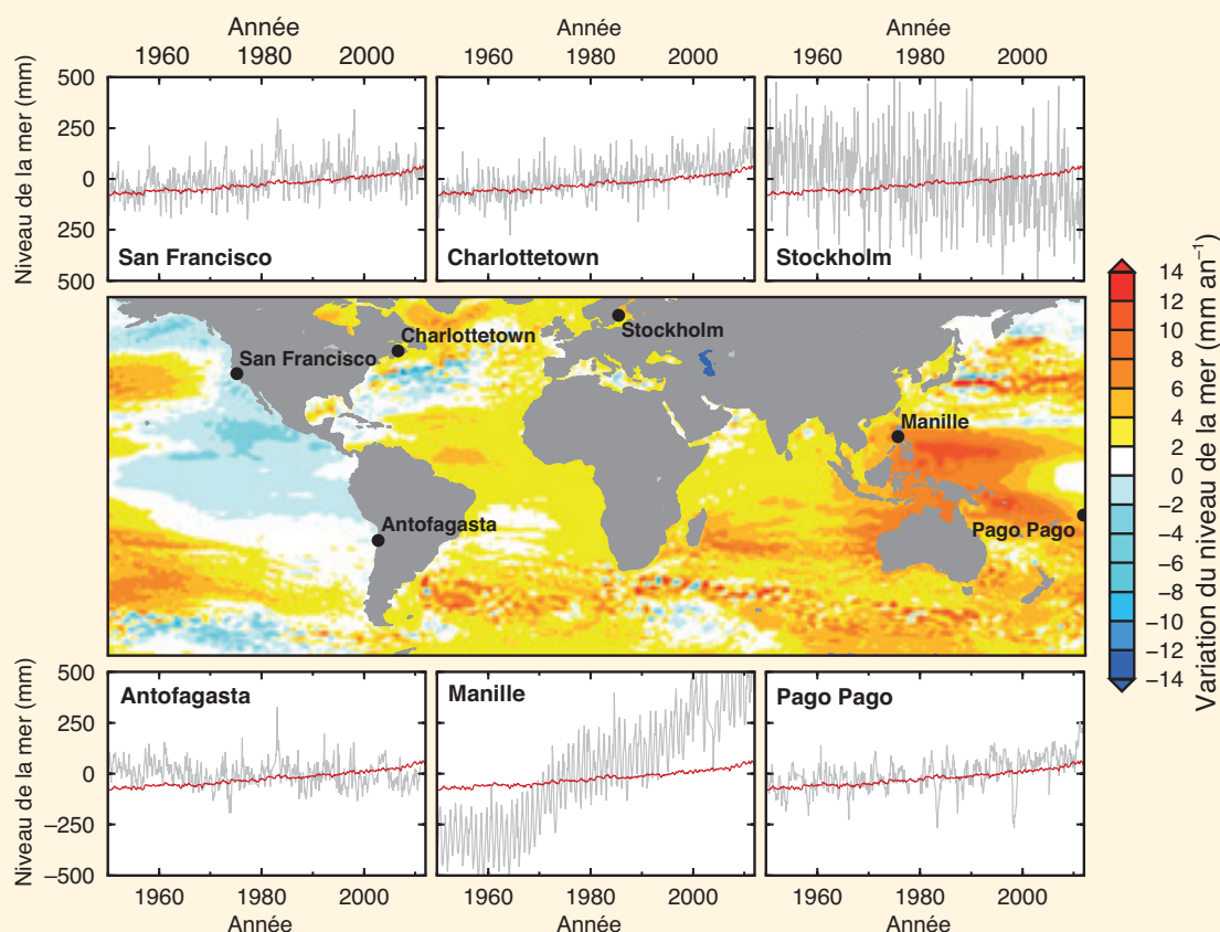
FAQ13.1 - Figure 1 | Carte des taux de variation de la hauteur de la surface des mers (niveau de la mer géocentrique) pour la période 1993–2012, établie à partir de données d'altimétrie satellitaire. La carte indique également les données de variation du niveau relatif de la mer (lignes en gris) relevées par des stations marégraphiques entre 1950 et 2012. Une estimation (en rouge) de la variation du niveau moyen mondial de la mer figure également (en rouge) avec chaque série chronologique de données des marégraphes pour comparaison. Les oscillations à court terme relativement importantes du niveau local de la mer (lignes en gris) sont imputables à la variabilité naturelle du climat décrite dans le corps principal du texte. Par exemple, les importants écarts réguliers relevés à Pago Pago sont associés au phénomène El Niño-Oscillation australe.
