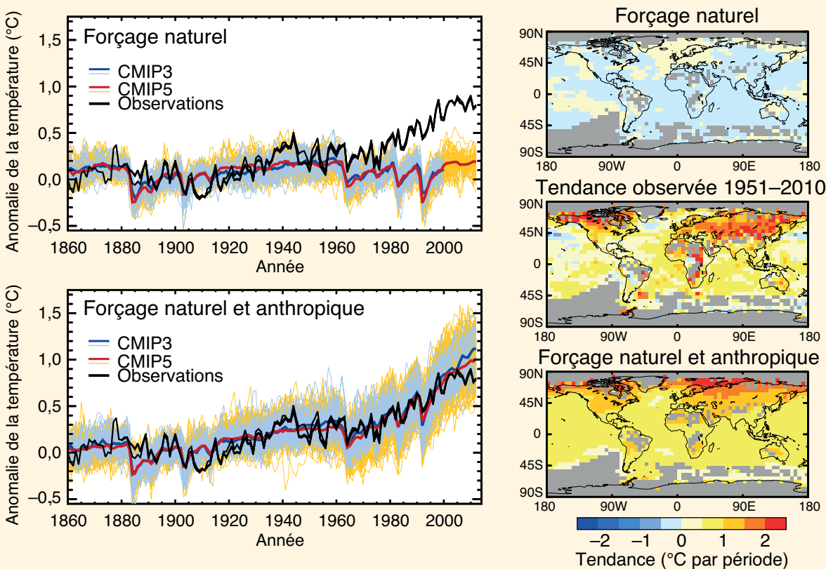
FAQ 10.1 - Figure 1 | (À gauche) Séries chronologiques de l'évolution des températures moyennes mondiales et annuelles en surface de 1860 à 2010. Le graphique en haut à gauche présente les résultats de deux ensembles de modèles climatiques basés uniquement sur les forçages naturels, indiqués par les fines lignes en bleu et jaune; les moyennes d'ensemble des variations de température sont indiquées par les lignes bleue et rouge épaisses. Les lignes noires indiquent trois estimations observationnelles différentes. Le graphique en bas à gauche présente des simulations provenant des mêmes modèles, mais intégrant à la fois le forçage naturel et les changements anthropiques de concentration des gaz à effet de serre et des aérosols. (À droite) Configurations spatiales des tendances locales de la température en surface de 1951 à 2010. Le graphique du haut présente la configuration des tendances données par un grand ensemble de simulations de la Phase 5 du Projet de comparaison de modèles couplés (CMIP5) et résultant uniquement des forçages naturels. Le graphique du bas présente les tendances d'un ensemble de simulations correspondantes, résultat des forçages naturels et anthropiques. Le graphique du milieu présente la configuration des tendances observées sur la même période à partir du jeu de données HadCRUT4.
