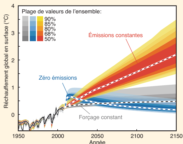
FAQ 12.3 - Figure 1 | Projections fondées sur le modèle MAGICC (Modèle d'évaluation du changement climatique induit par les gaz à effet de serre) du bilan énergétique et du cycle du carbone pour une composition constante de l'atmosphère (forçage constant, en gris), des émissions constantes (en rouge) et des émissions futures à zéro (en bleu), à partir de 2010, avec des estimations de l'incertitude. Figure adaptée de Hare et Meinshausen (2006), fondée sur l'étalonnage d'un modèle climatique simple du cycle du carbone avec tous les modèles de la Phase 3 du Projet de comparaison de modèles couplés (CMIP3) et du projet de comparaison des modèles couplés climat-cycle du carbone (C4MIP) (Meinshausen et al. , 2011a; Meinshausen et al. , 2011b). Les résultats sont fondés sur une simulation transitoire complète partant de l'ère préindustrielle et utilisant toutes les composantes du forçage radiatif. La fine ligne noire et la zone ombrée dénotent le réchauffement observé et l'incertitude.
