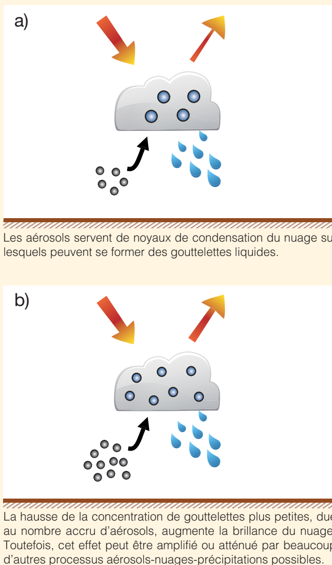
FAQ 7.2 - Figure 2 | Aperçu des interactions entre les aérosols et les nuages et de leur incidence sur le climat. Nuage de l'étage inférieur a) non pollué et b) pollué.
